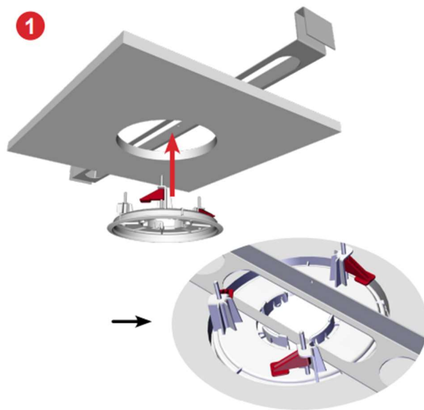
タイルブリッジの開口部のブラケットの向き
