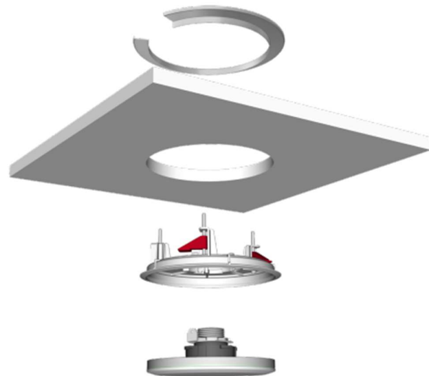
TCM-X-FM分解アセンブリ
